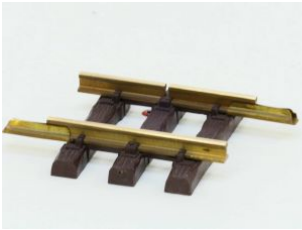
LGB 1008 W Ger. Unterbrechergleis, 82mm
