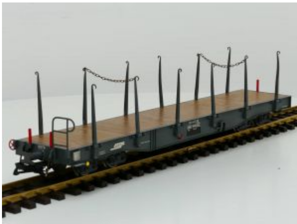
Scheba 1103.002.004 Vierachsiger Plattformwagen der RhB Rp-w 8278
